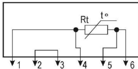
Четырехпроводная схема включения ТС
